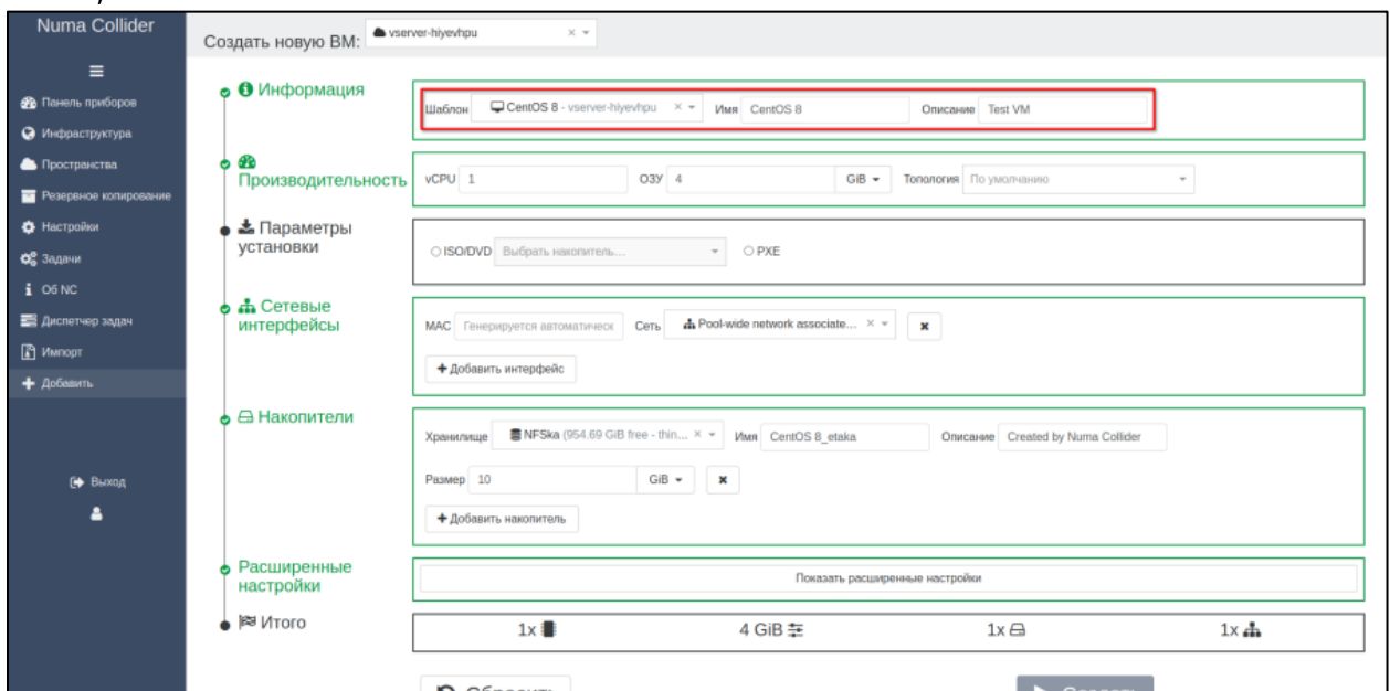
Рисунок 18 – Имя и описание виртуальной машины
