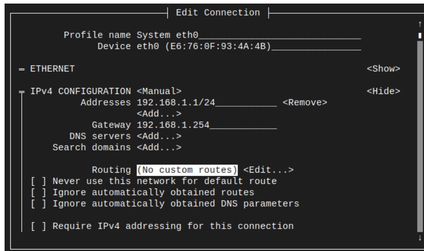
Рисунок 31 – Пример ввода статических параметров сети
