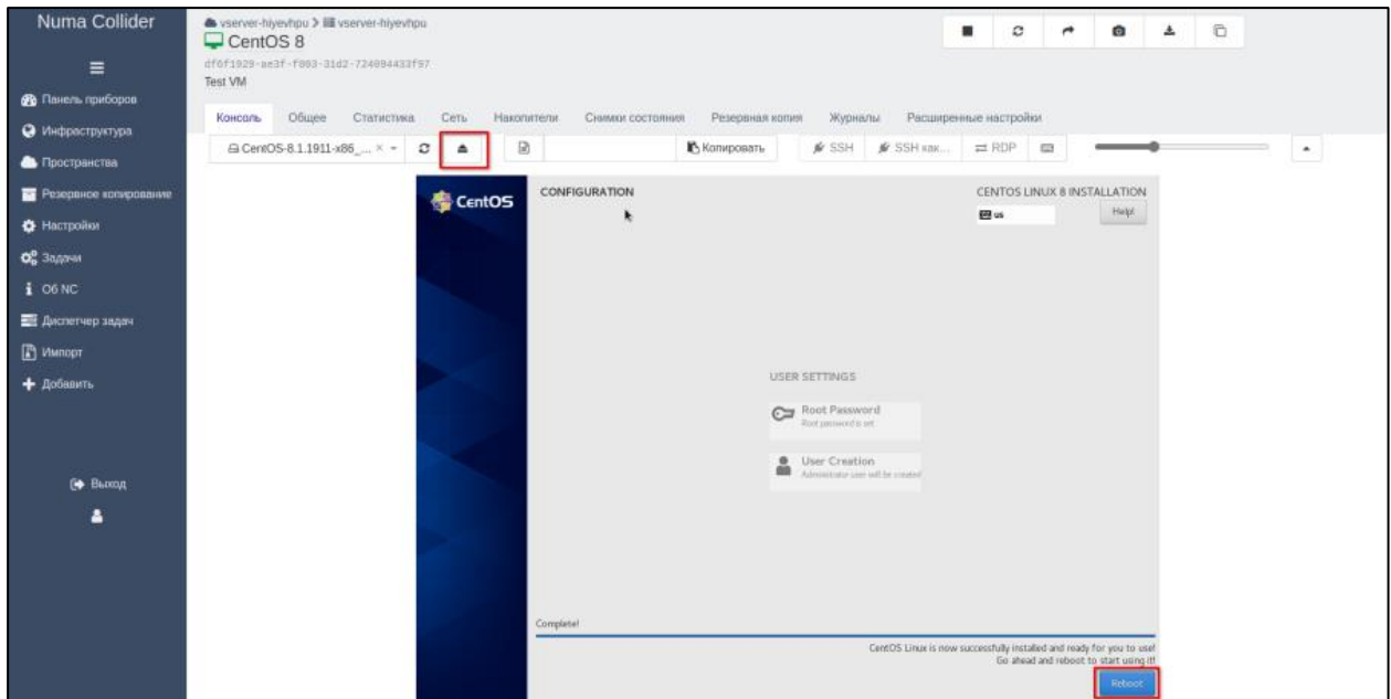
Рисунок 21 – Размонтирование образа
